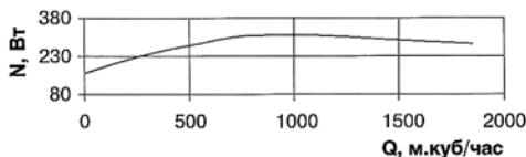
Акустические характеристики MER 315/1
