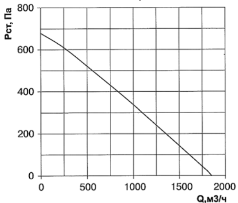
Технические данные вентиляторов MER 315/1
