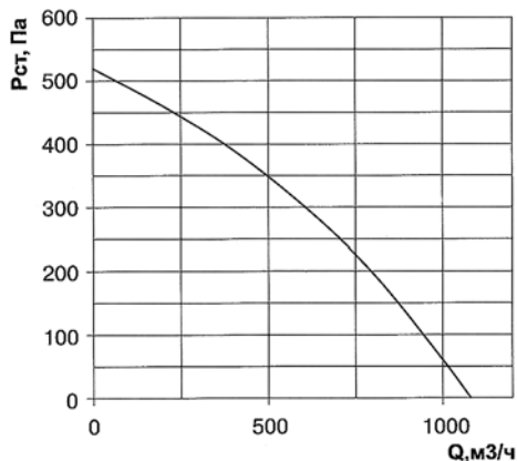
Технические данные вентиляторов MER 250/1
