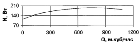
Акустические характеристики MER 250/1
