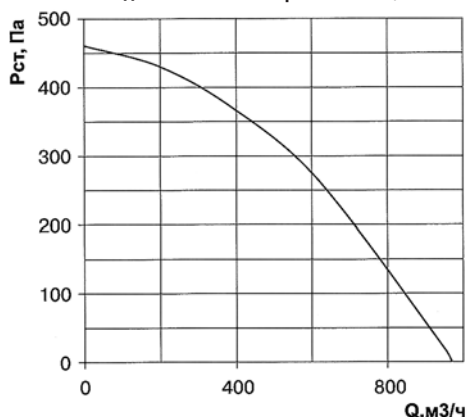
Технические данные вентиляторов MER 200/1
