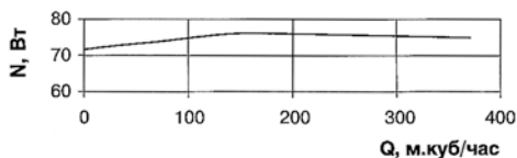
Акустические характеристики MER 125/1
