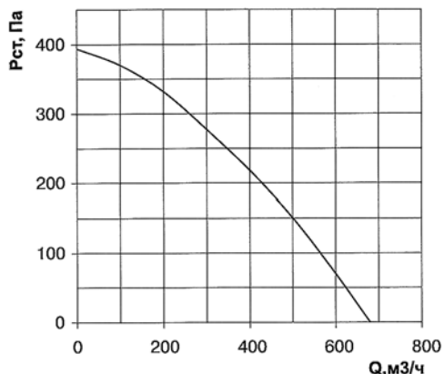
Технические данные вентиляторов MER 160/1
